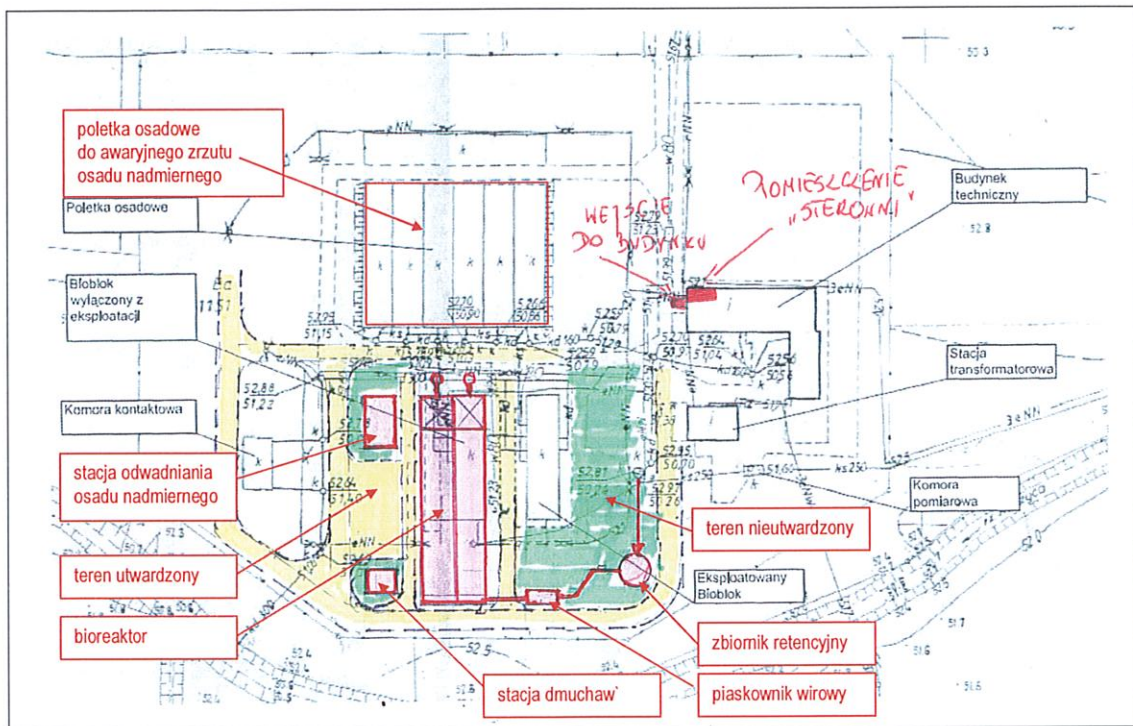
SZKIC KONCEPCYJNY PLANU ZAGOSPODAROWANIA TERENU
